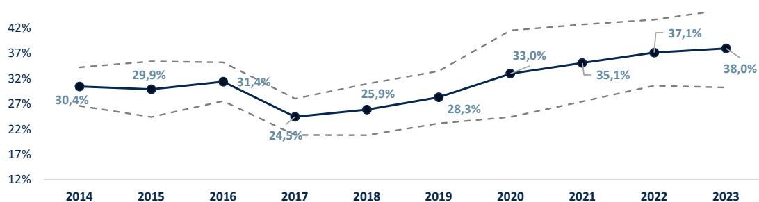
Evolution de la décote de holding moyenne et de son intervalle de confiance statistique à 95% entre 2014 et 2023
